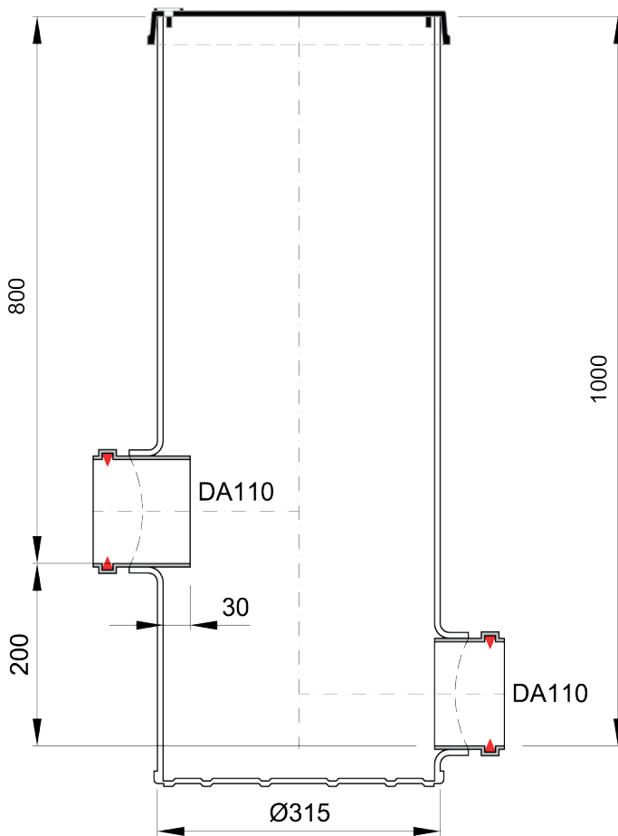
PVC - Probeentnahmeschacht DN 315 mit Gussdeckel A15, begehbar
